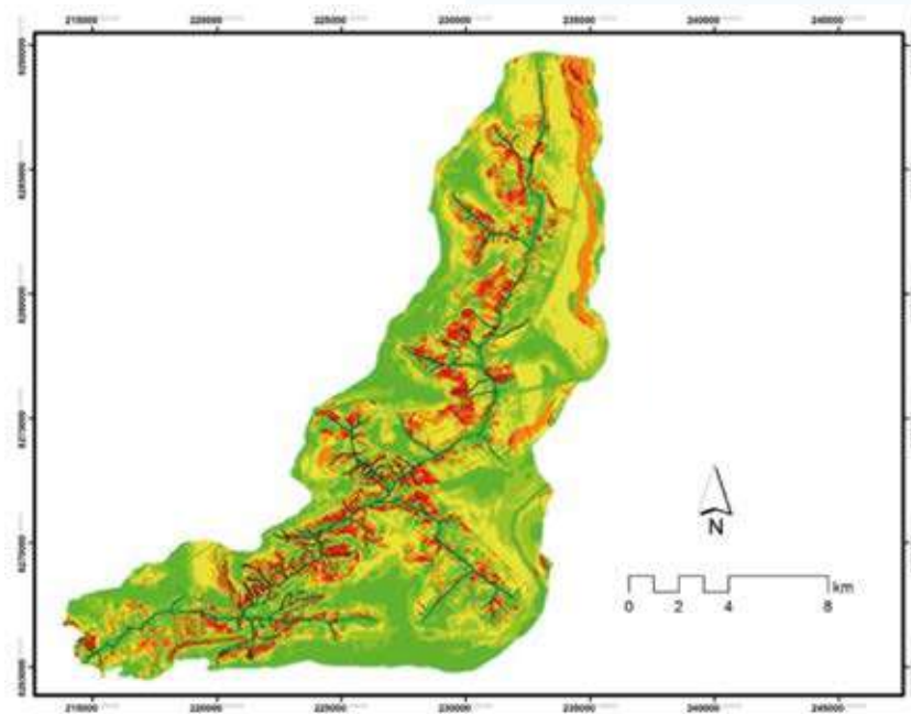
Figura 3. Mapa de erosão média anual da bacia do Ribeirão Pipiripau, calculada por meio da USLE + SIG Fonte: Chaves, 2012.
