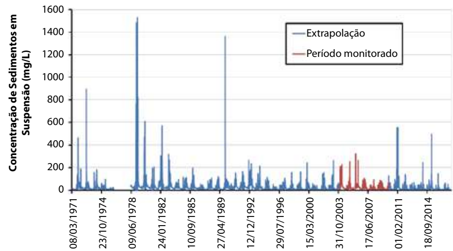
Figura 11. Série temporal estimada da concentração de sedimentos em suspensão na estação Frinocap DF-130 do Ribeirão Pipiripau
