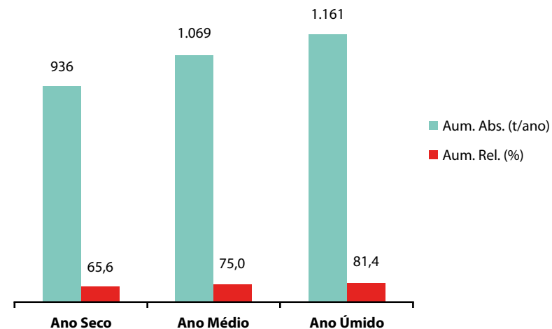
Figura 6. Estimativa da redução no aporte de sedimento ao exutório da bacia depois da implantação integral do PPA Fonte: Chaves, 2012.
