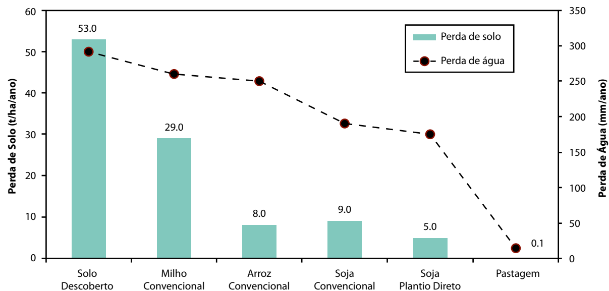
Figura 1. Perda de solo e de água em parcelas de monitoramento da enxurrada (calhas de Wischmeier) sob diferentes tipos de uso em um latossolo vermelho escuro do Cerrado Fonte: Dedecek et al., 1986.
