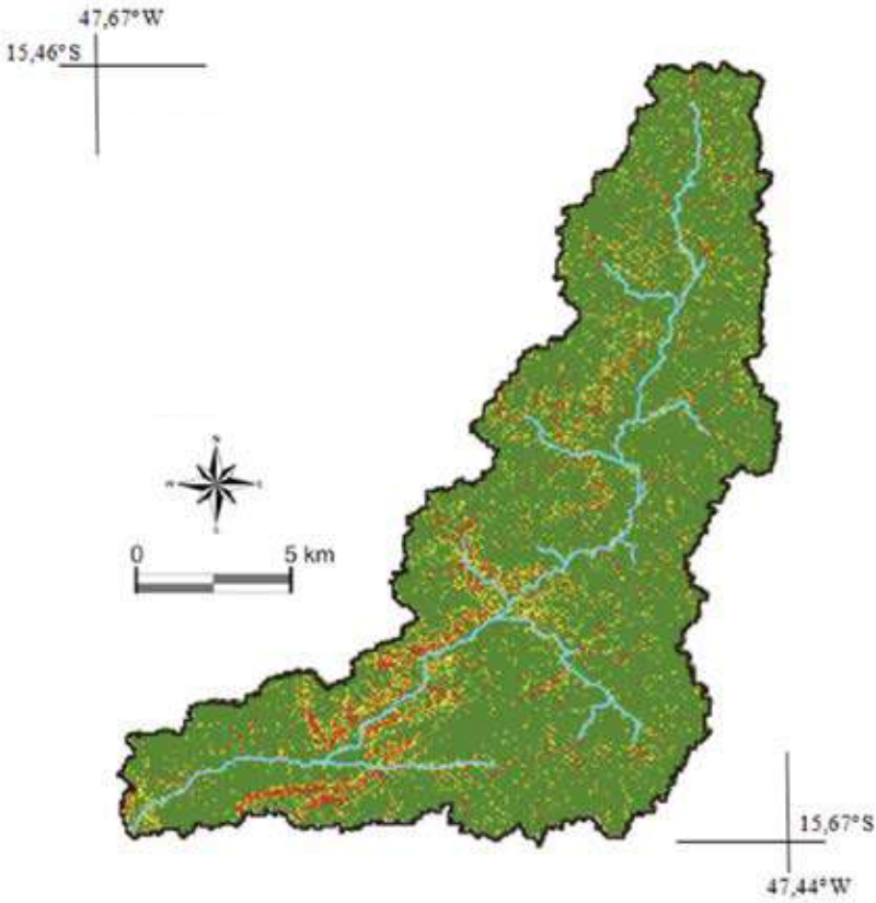
Figura 4. Mapa de susceptibilidade à erosão da bacia do Ribeirão Pipiripau, em células de 30 m Fonte: Lima et al., 2013b.
