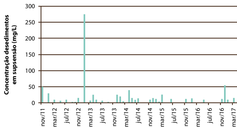
Figura 9. Dados de medições da concentração de sedimentos em suspensão realizadas entre 2011 e 2017 na estação Montante Canal do Ribeirão Pipiripau
