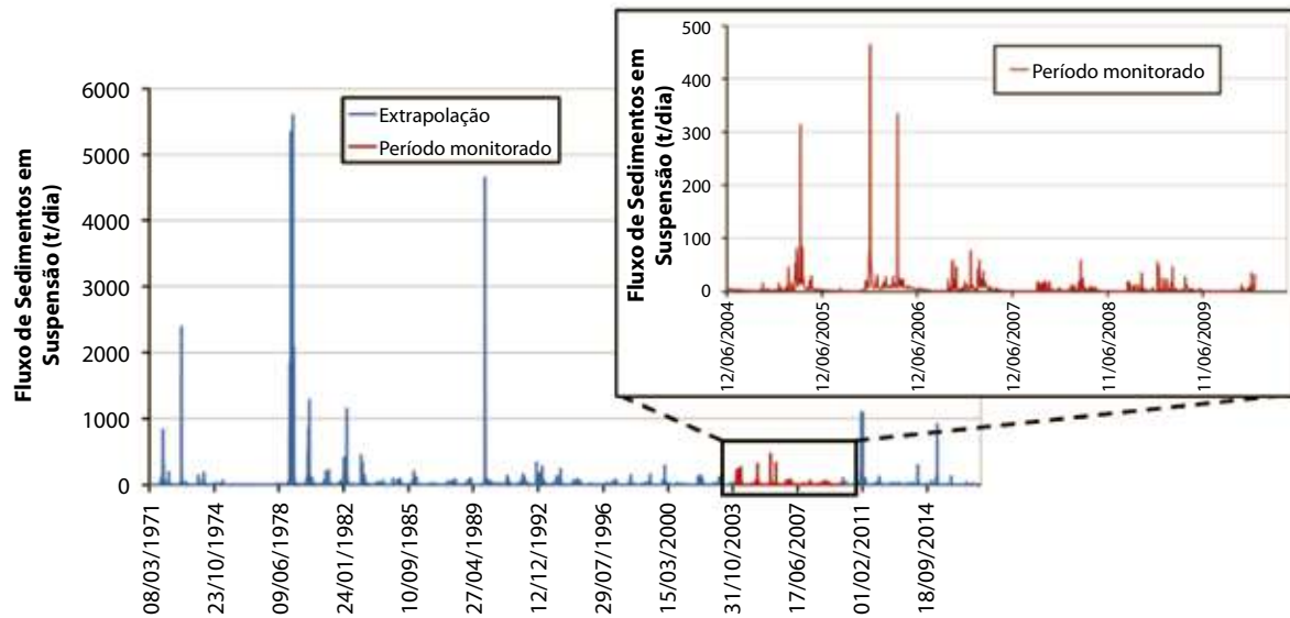
| Figura 12. Série temporal estimada do fluxo de sedimentos em suspensão na estação Frinocap DF-130 do Ribeirão Pipiripau
